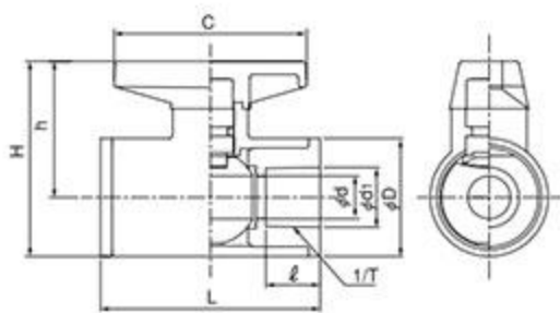
●TS承口 ( 13A×15A )
