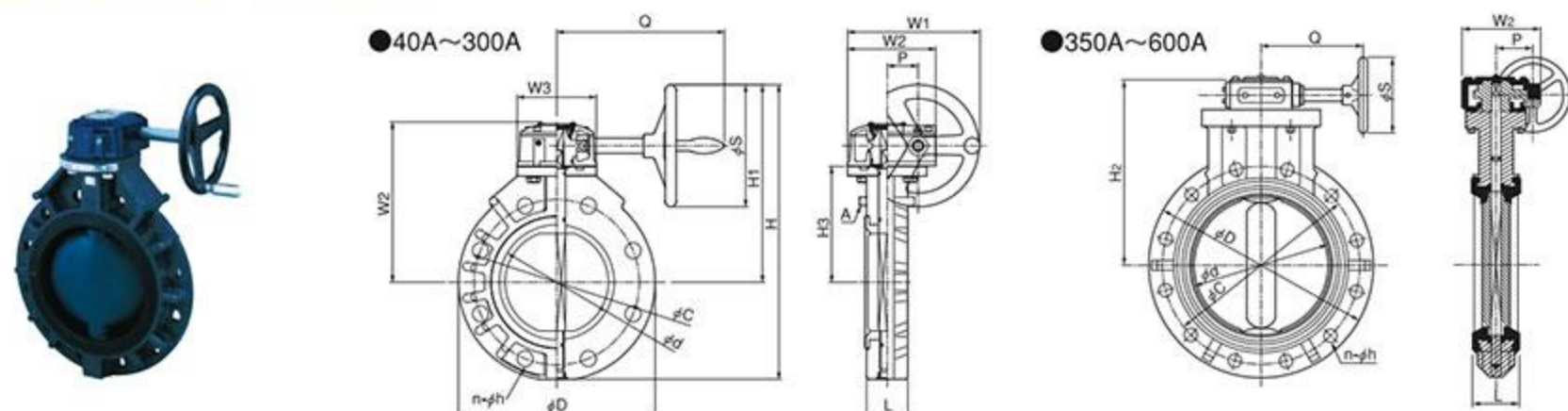
尺寸表40A~300A
