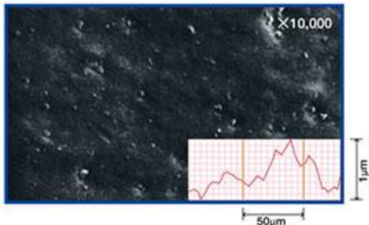
普通PVC管道
