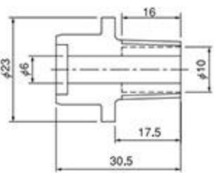
●外牙螺纹接口 ( R1/2 )
