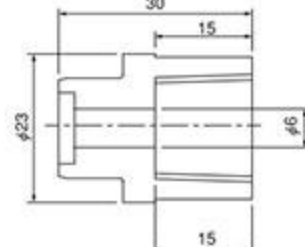
●内牙螺纹接口 ( RC1/4×3/8 )
