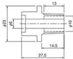
●外牙螺纹接口 ( R1/4 · 3/8 )
