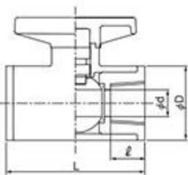
●螺纹接口 ( 13A×15A )
