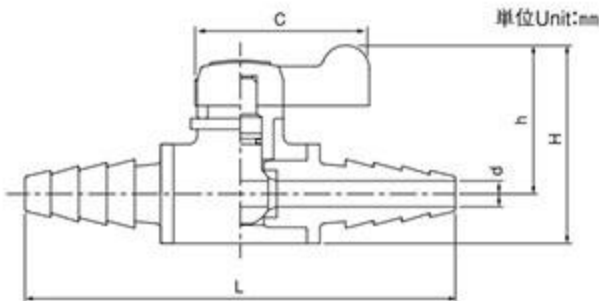
●软管接口×软管接口 ( 6A )
